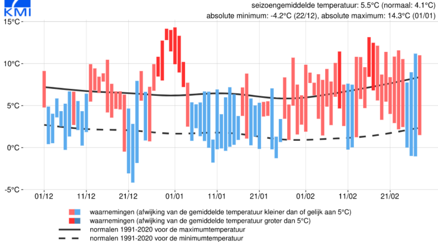
Dagelijkse temperatuurverschillen, Ukkel, winter 2022
